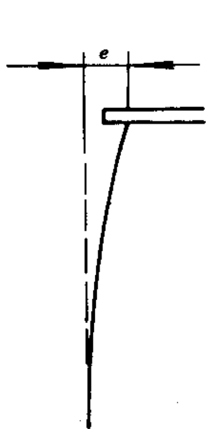
图 7 桌面水平耐久性试验位移值测量方法
